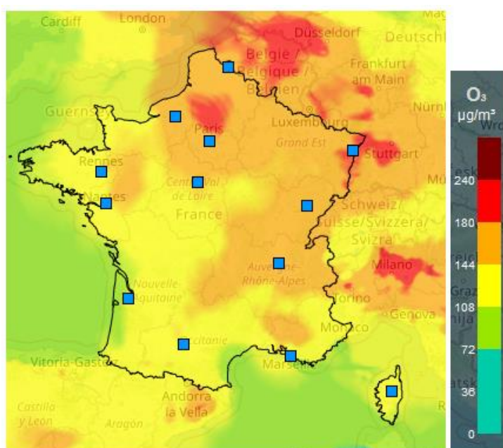
carte prévoir de concentration en Ozone pour la journée du 31 juillet.
