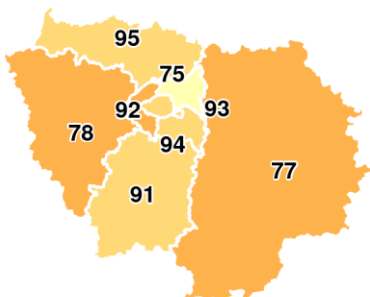
Taux d'Incidence
