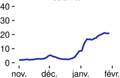
Positivité
