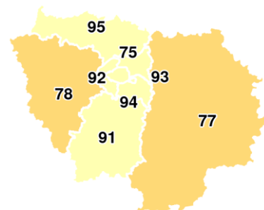
Alarmes
