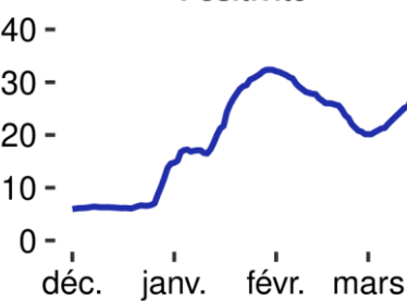
Positivité
