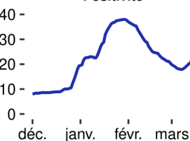
Positivité
