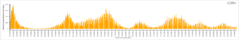
Nombre de cas de COVID-19 nouvellement admis en réanimation par jour, en France, du 19 mars 2020 au 9 septembre 2022, données SI-VIC
