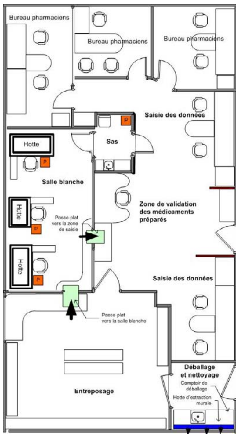
FIGURE 9 Exemple d'aménagement d'une pharmacie d'oncologie ayant un fort volume de préparation
